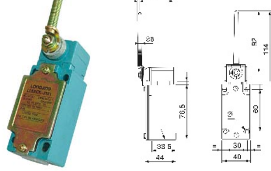
LL8XCK-J181 LL8XCK-J281 四回路双断型
